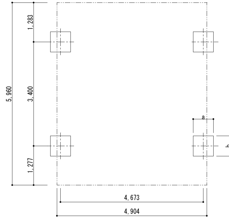
■ 基礎配置図
